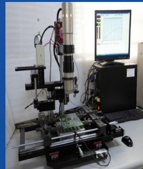
BGA 返修設備
